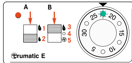
Bedienteil der Gasheizung
