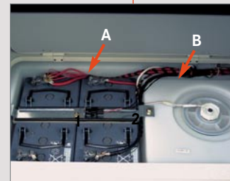
12-V-Zusatzbatterien (A) Reinigungsöffnung Frischwassertank (B)
